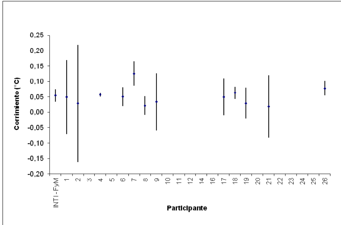
Gráfico 1: Corrimientos a -30°C
