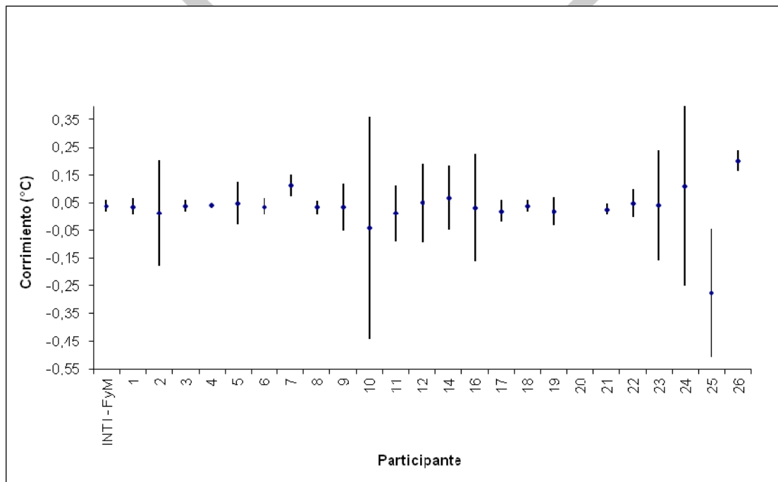
Gráfico 2: Corrimientos a 0°C
