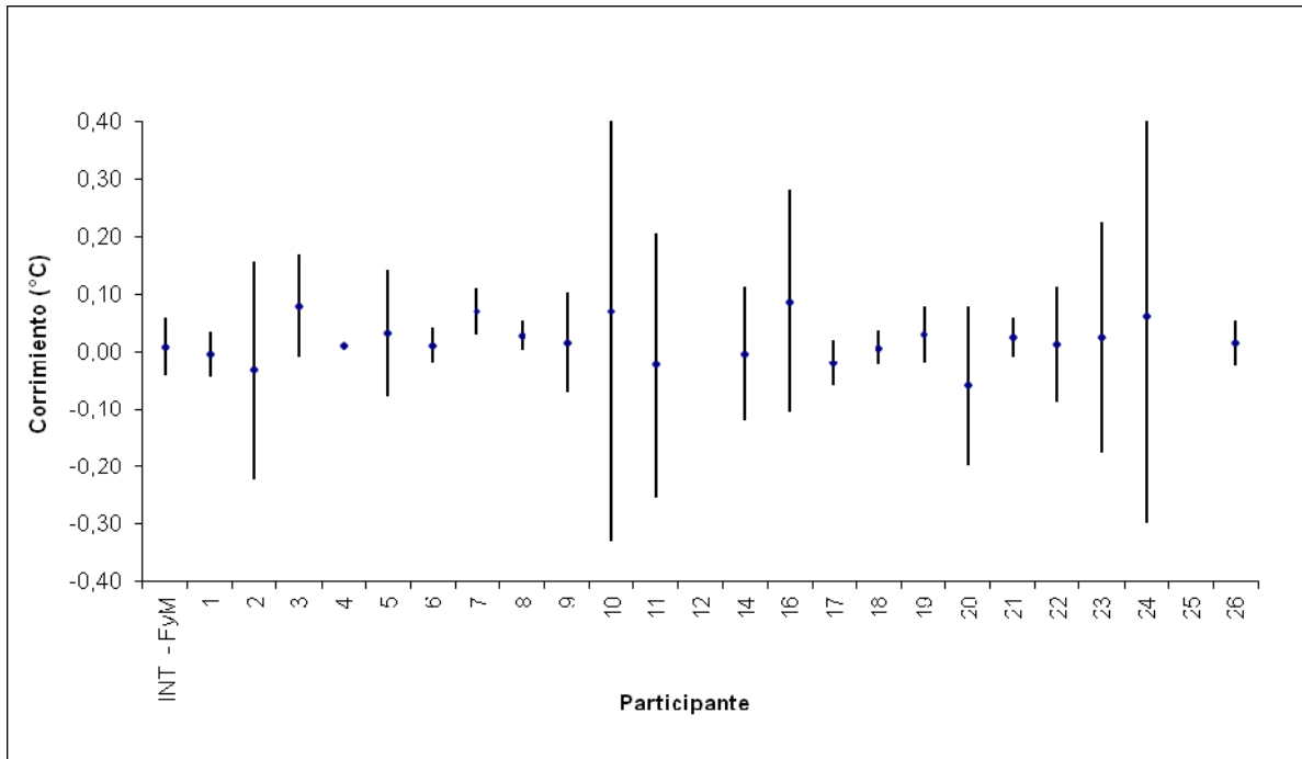
Gráfico 4: Corrimientos a 90°C
