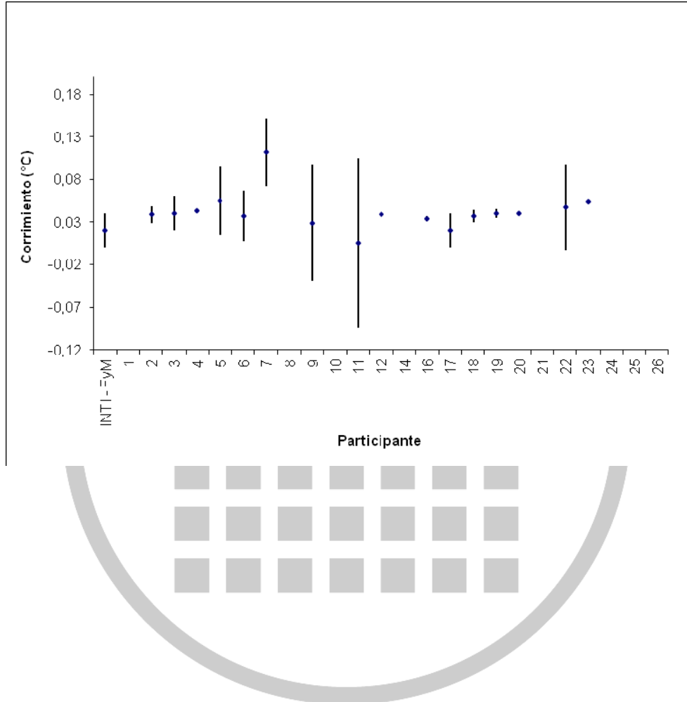
Gráfico 8 – Corrimientos en el punto de hielo
