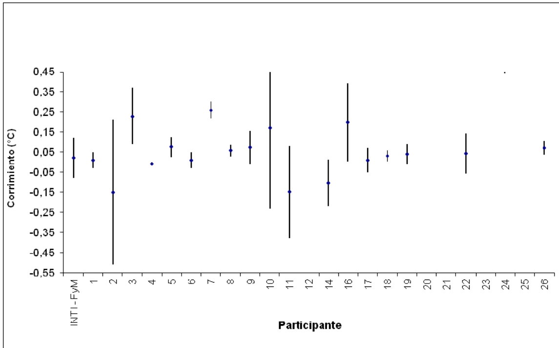
Gráfico 6: Corrimientos a 200°C
