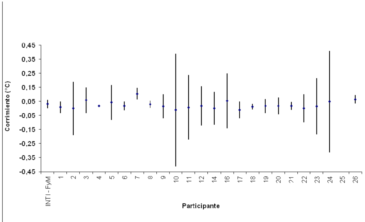
Gráfico 3: Corrimientos a 40°C
