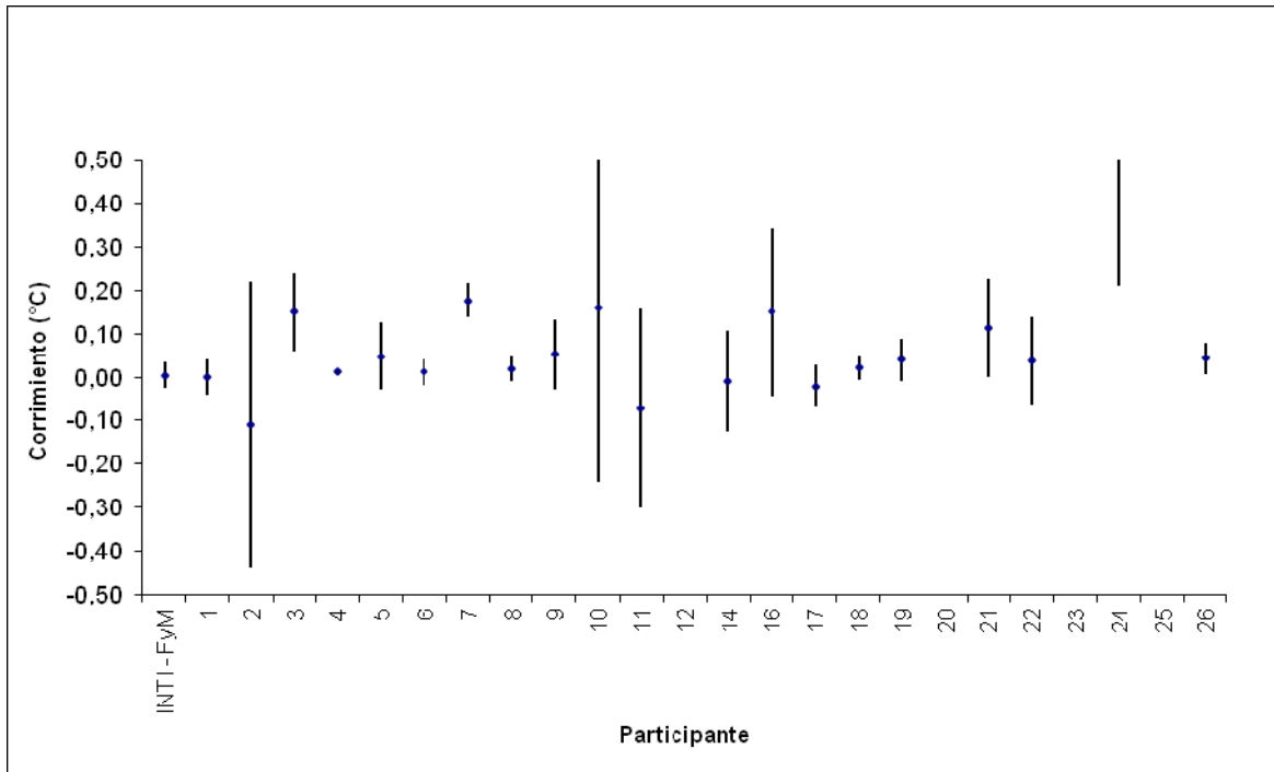
Gráfico 5: Corrimientos a 150°C
