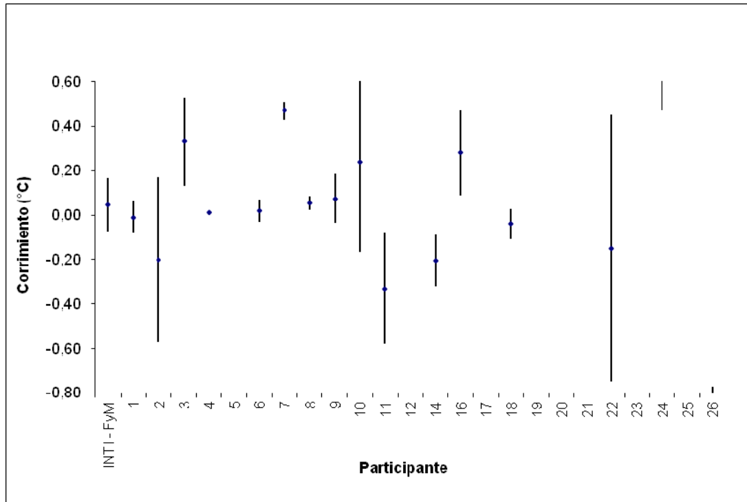
Gráfico 7: Corrimientos a 300°C
